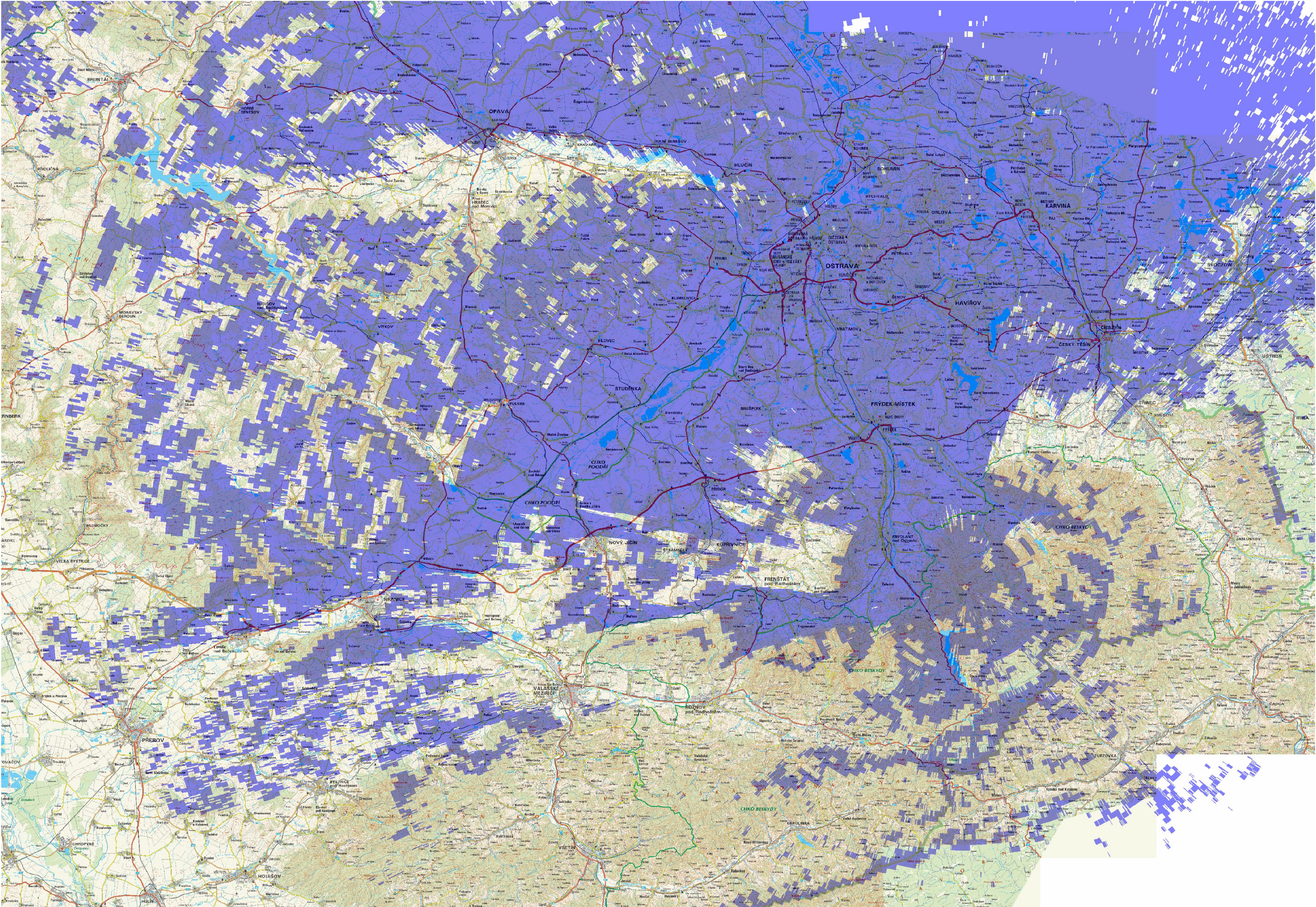
pokrytí vysílače Frýdek Místek - Lysá hora LP5 kW, intenzita pole 65 dBu/m, pokryto 1 057 304 obyvatel
